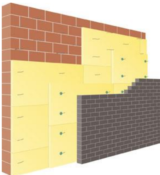
Fig. 1: Pose multicouche
